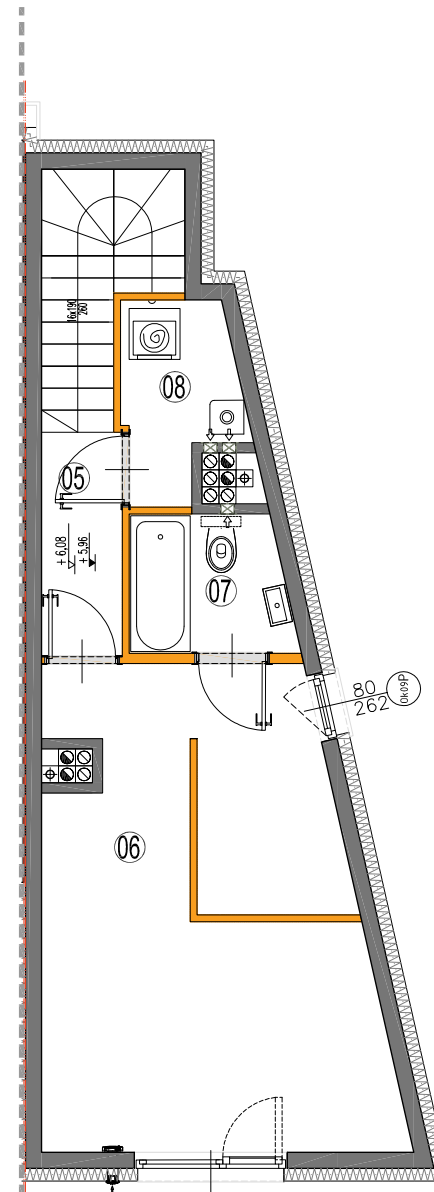
RZUT PIĘTRA +2
