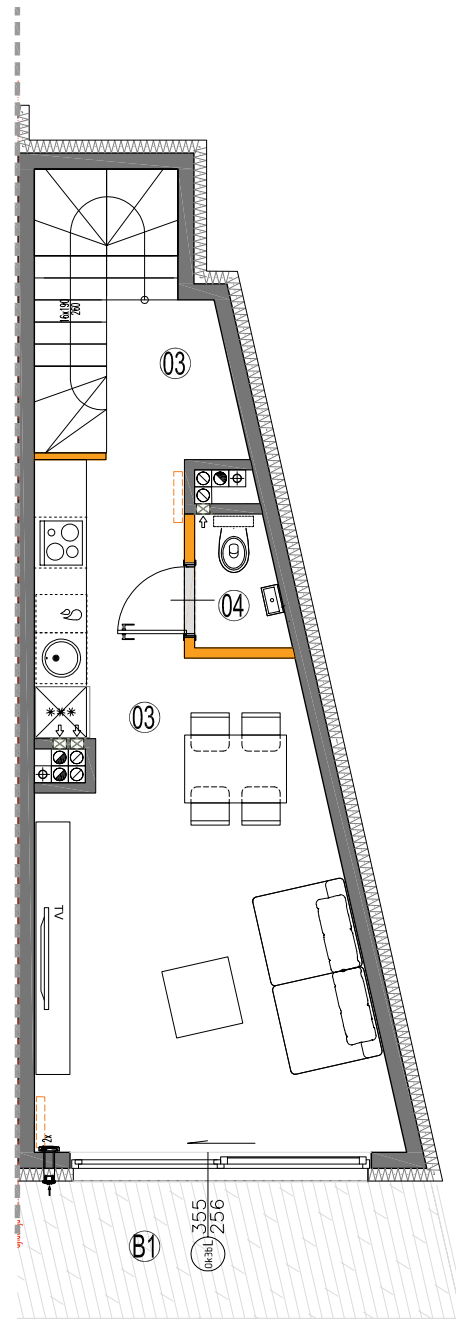
RZUT PIĘTRA +1
